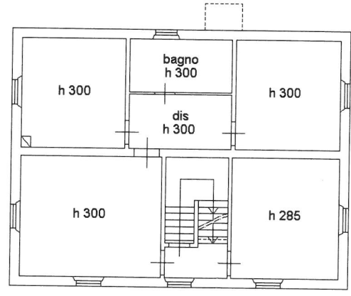
PIANO SECONDO
